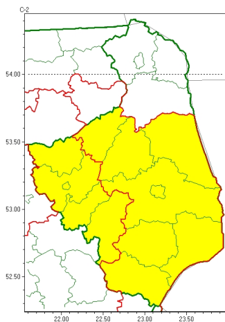
Opady marznące 2022-11-21 10:31
